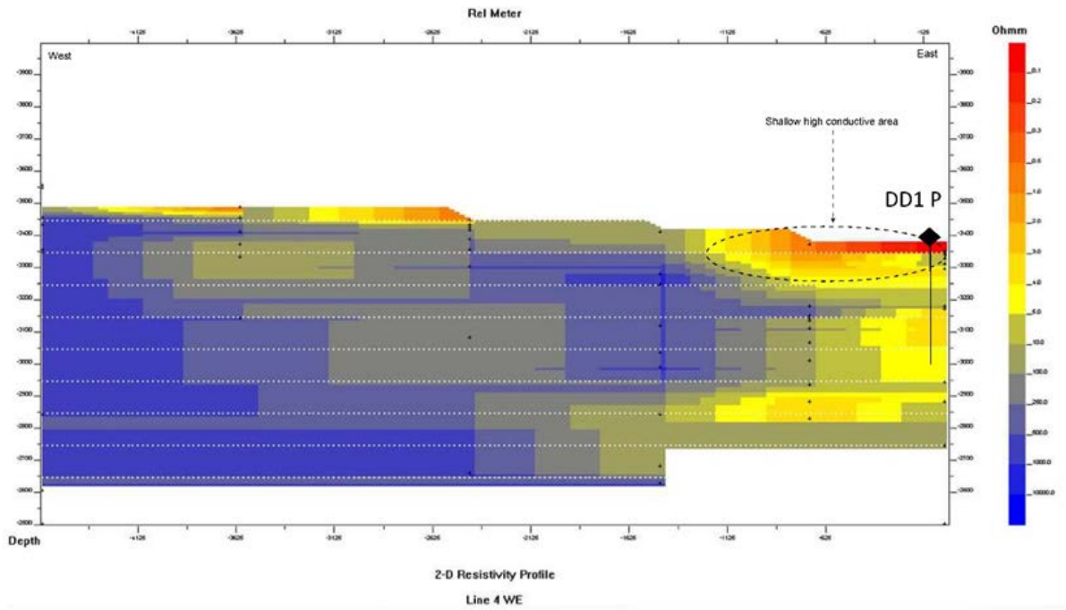
Figure 2. CSAMT Results Line 4
